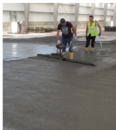
Vibroépandage magic screed
